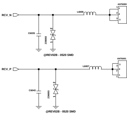
RCV CONTACT
